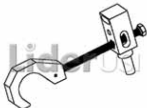
Código: G019 Descrição: Gabarito - Regulação da pinça do cilindro armazém
